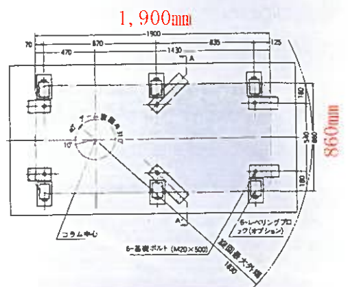
●基礎図
