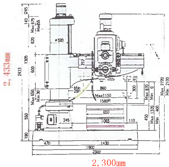
●外形図
